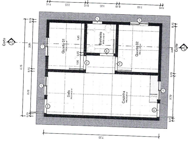
3 Planta Baixa 1:50
